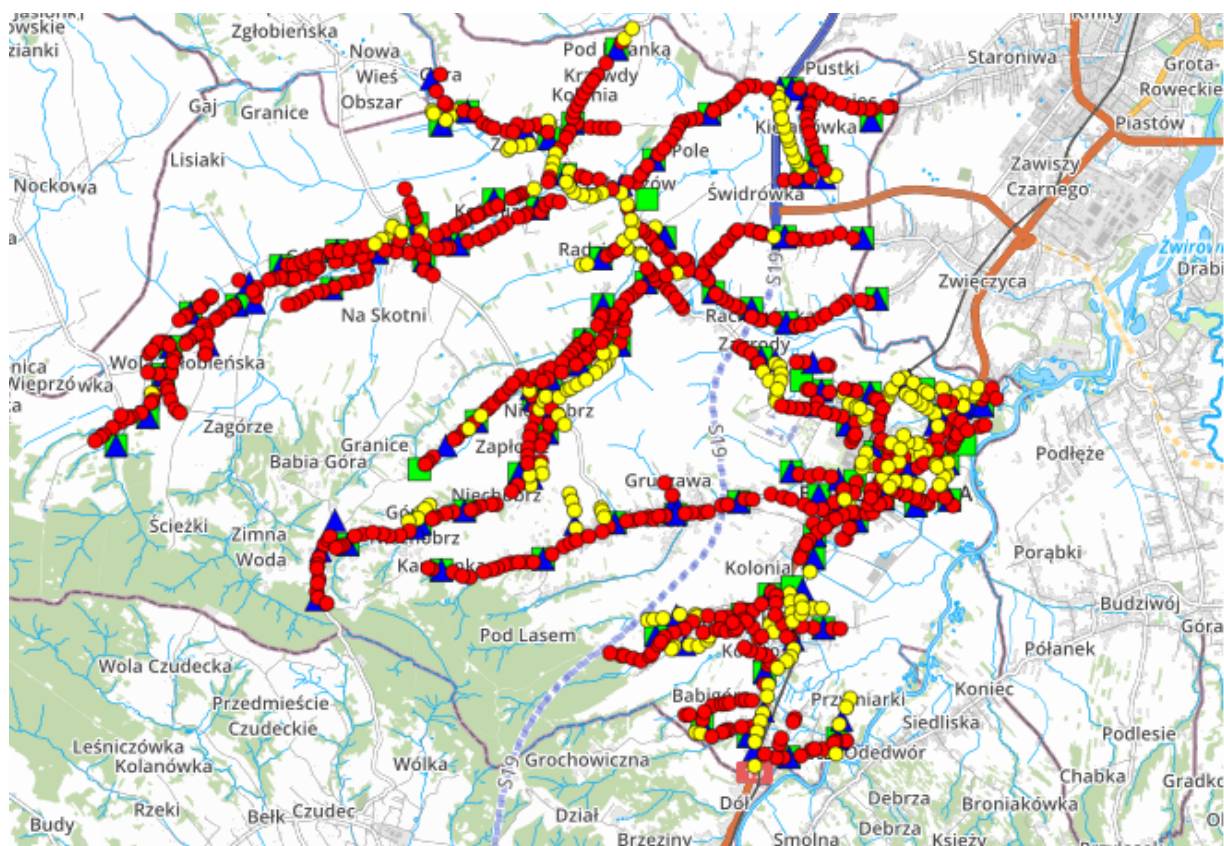
Rysunek 1: Sieć oświetlenia drogowego na terenie Gminy Boguchwała [kolor czerwony PGE, kolor żółty Gmina]
